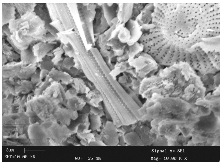
Rysunek 3. Fragmenty skoruppek Melosira sp. (po lewej) i Stephanodiscus sp. (po prawej) w próbkach osadów dennych zbiornika Dobromierz
