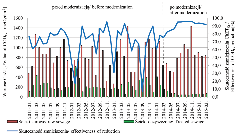
Rysunek 4. Zestawienie wartości \text{ChZT}_{\text{Cr}} ścieków surowych i oczyszczonych na tle skuteczności jego zmniejszenia przed i po modernizacji
