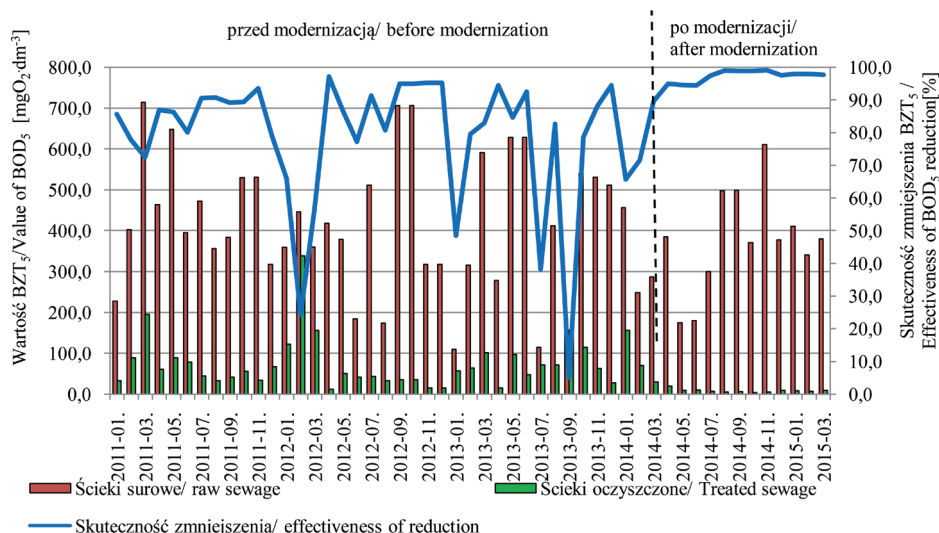
Rysunek 3. Zestawienie wartości BZT_5 ścieków surowych i oczyszczonych na tle skuteczności jego zmniejszenia przed i po modernizacji
