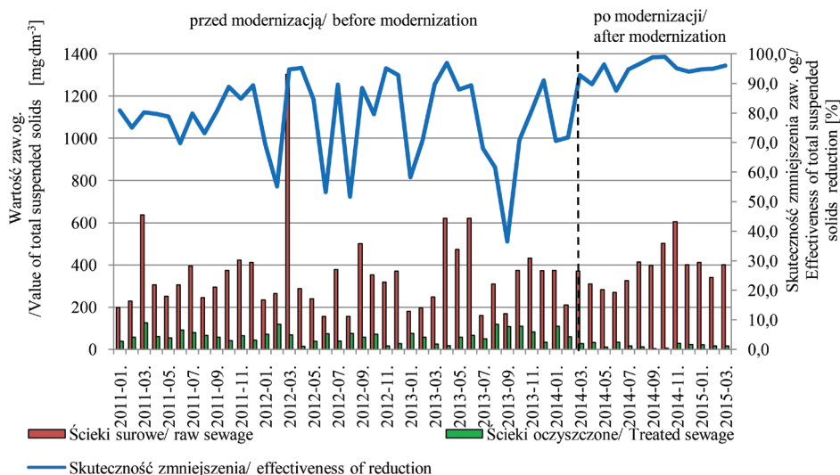
Rysunek 5. Zestawienie wartości zawiesiny ogólnej w ściekach surowych i oczyszczonych na tle skuteczności jej zmniejszenia przed i po modernizacji
