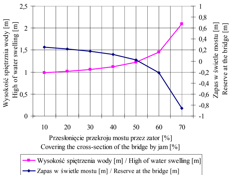
Rysunek 4. Wysokość spiętrzenia i zapas w świetle mostu w km 27+500 potoku Wieprzówka w przypadku powstania zatoru z rumoszu drzewnego
