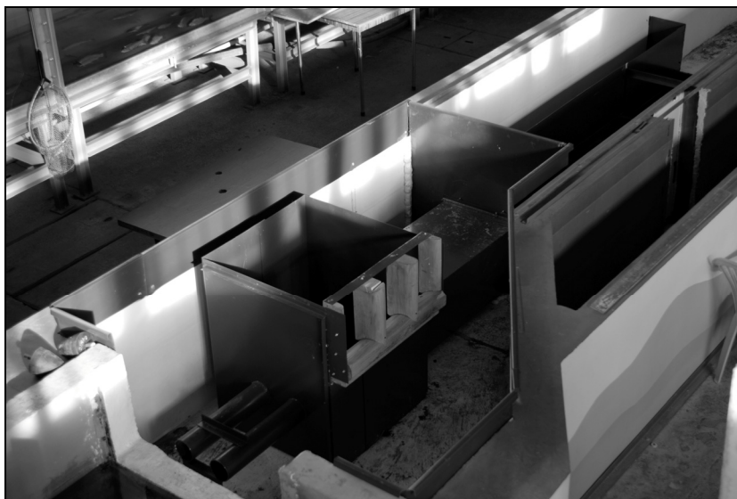
Rysunek 2. Stanowisko badawcze Figure 2. Laboratory flume
