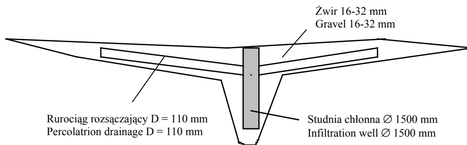
Rysunek 1. Schemat rowu infiltracyjnego z drenażem rozszczajającym oraz studnią chłonną
