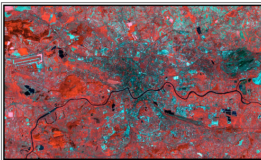
Rysunek 2. Kompozycja barwna utworzona z kanałów 4, 3, 2 satelity Landsat-7 Figure 2. Color composition made of 4,3,2 chanelns of satellite Landsat-7
