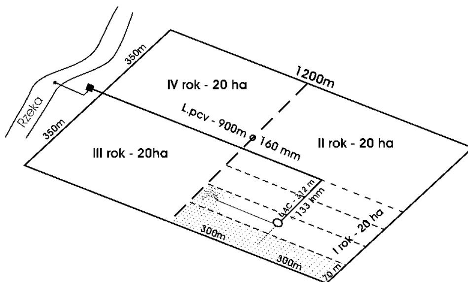
Rysunek 7. Przykład nawadniania plantacji – powierzchnia 20 ha
