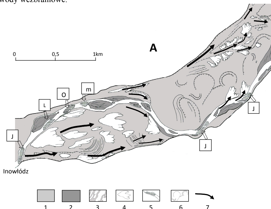
Rysunek 4. Morfologia tarasu zalewowego Pilicy poniżej Inowódza: 1 – powierzchnia tarasu zalewowego rzeki meandrującej, 2 – taras współczesny, 3 – wielkoskalowe odsypy (rys. 5), 4 – stożki napływowe (glify krewasowe), 5 – trudno rozmywane progi w korycie: J – piaskowce jury, m – utwory morenowe, L – residualne bruki, o – osady organiczne, 6 – ślady przemieszczania się koryta, starorzecza i rynny erozyjne, 7 – kierunki przepływu wód wezbraniowych
