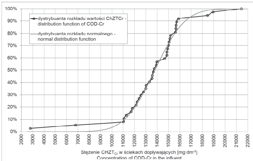
Rysunek 6. Dystrybuanta rozkładu wartości ChZTCr na dopływie oczyszczalni oraz rozkładu normalnego o najmniejszym błędzie średniokwadratowym aproksymacji wartości ChZTCr Figure 6. Distribution function of COD-Cr in the effluent flow and a normal distribution with a minimum mean square error of approximation value of COD-Cr
