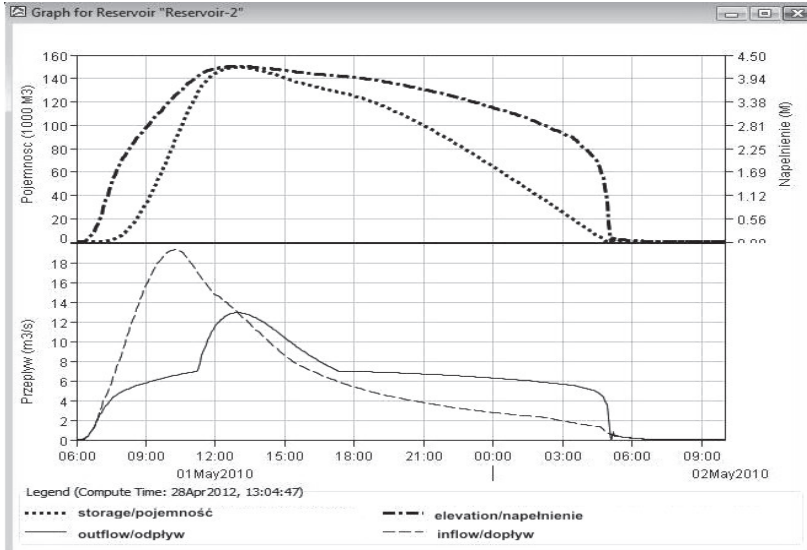
Rysunek 3. Wynik symulacji pracy zbiornika Biezanów w wariacie II dla opadu o czasie trwania 1 h.
