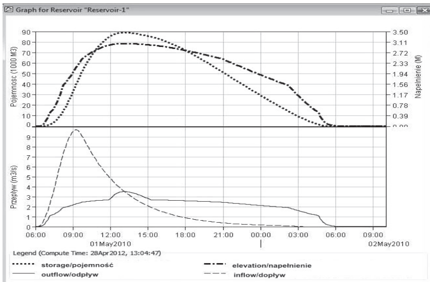
Rysunek 4. Wynik symulacji pracy zbiornika Malinówka w wariacie II dla opadu o czasie trwania 1 h.
