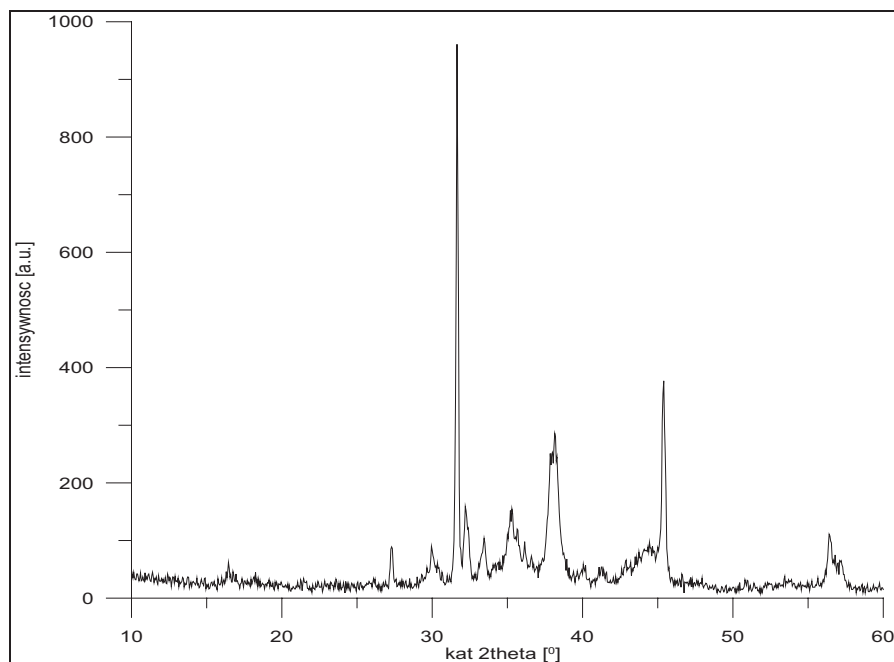
Rysunek 8. Dyfraktogram XRD cząstek magnetycznych otoczonych nanosrebrzem i stabilizowanych 3 % r-rem gumy arabskiej po 120 min.
