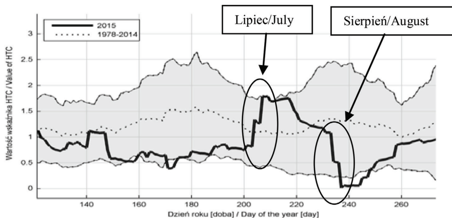
Rysunek 4. Wpływ incydentów opadowych w 2015 roku na wartości współczynnika HTC – Toruń, centralna Polska .
