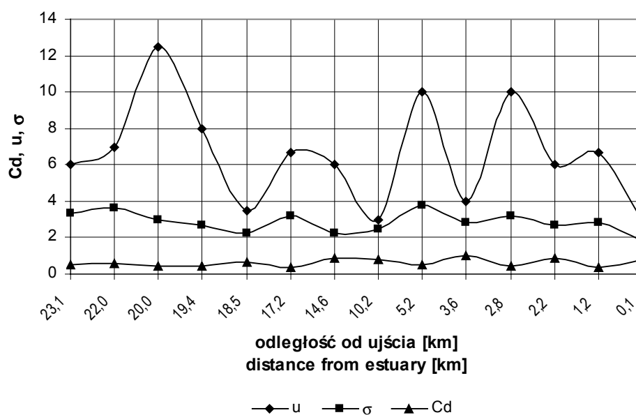
Rysunek 5. Zmienność wskaźników charakterystycznych rumowiska wzdłuż potoku Słomka
