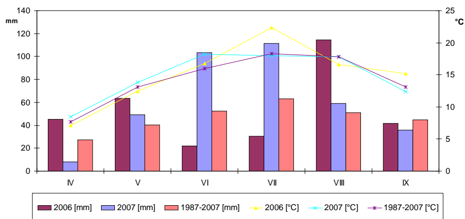
Rysunek 1. Opady atmosferyczne [mm] i temperatura powietrza [°C] w Kruszynie Krajeńskim w latach 2006 i 2007 Figure 1. Precipitation [mm] and temperature [°C] at Kruszyn Krajeński in the years 2006 and 2007
