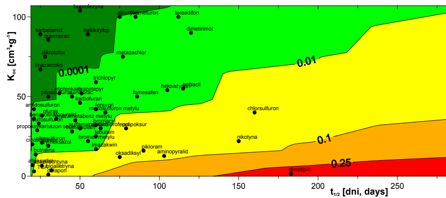
Rysunek 3. Zależność średniej podatności zlewni ( AF_{sr} ) od czasu połowicznego rozkładu i współczynnika sorpcji Figure 3. Mean vulnerability of the catchment area ( AF_{sr} ) as a function of t_{1/2} and sorption coefficient K_{oc}
