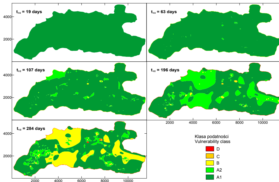
Rysunek 2. Mapy podatności przy współczynniku sorpcji K_{oc} = 107 \text{ cm}^3 \cdot \text{g}^{-1} dla różnych czasów połowicznego rozkładu Figure 2. Maps of groundwater vulnerability for K_{oc} = 107 \text{ cm}^3 \cdot \text{g}^{-1} and various half-life time
