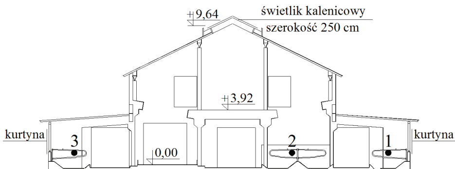
Rysunek 1. Rozmieszczenie punktów pomiarowych prędkości i temperatury powietrza (1-4) w oborze w Kobylanach: a – rzut, b – przekrój I-I
