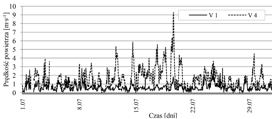
Rysunek 3. Średnio godzinowe prędkości wiatru (V4) i powietrza wentylacyjnego (V1) na pierwszym stanowisku pomiarowym w lipcu 2012
